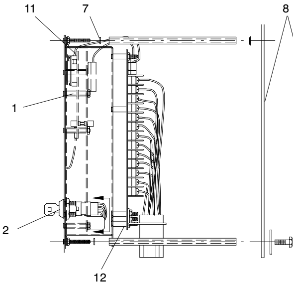
View A-A
