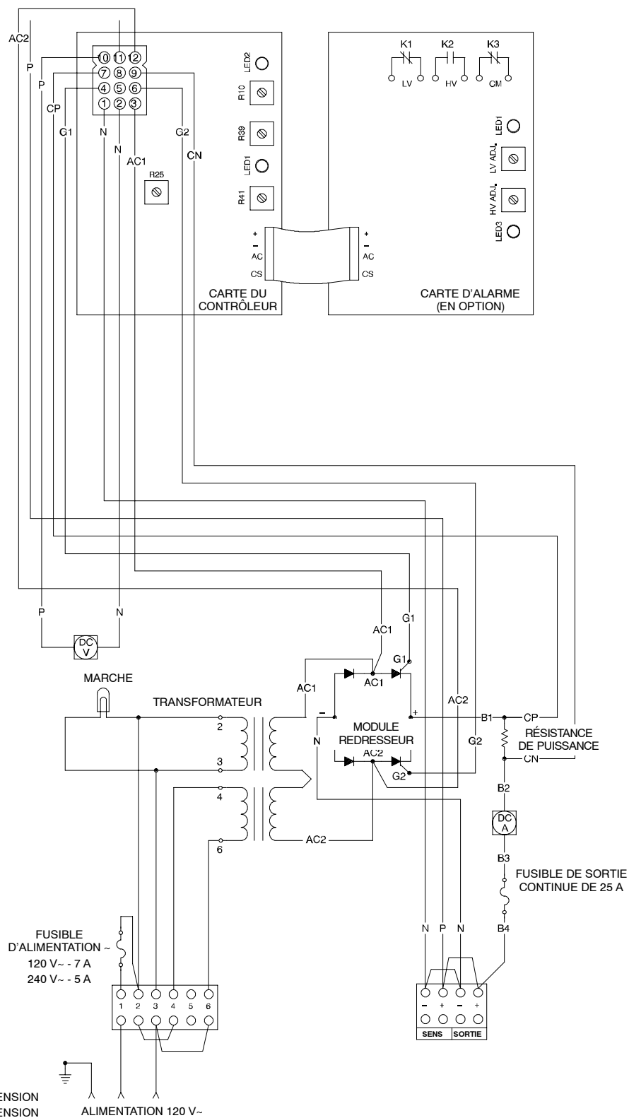
Schéma de câblage 233968A
