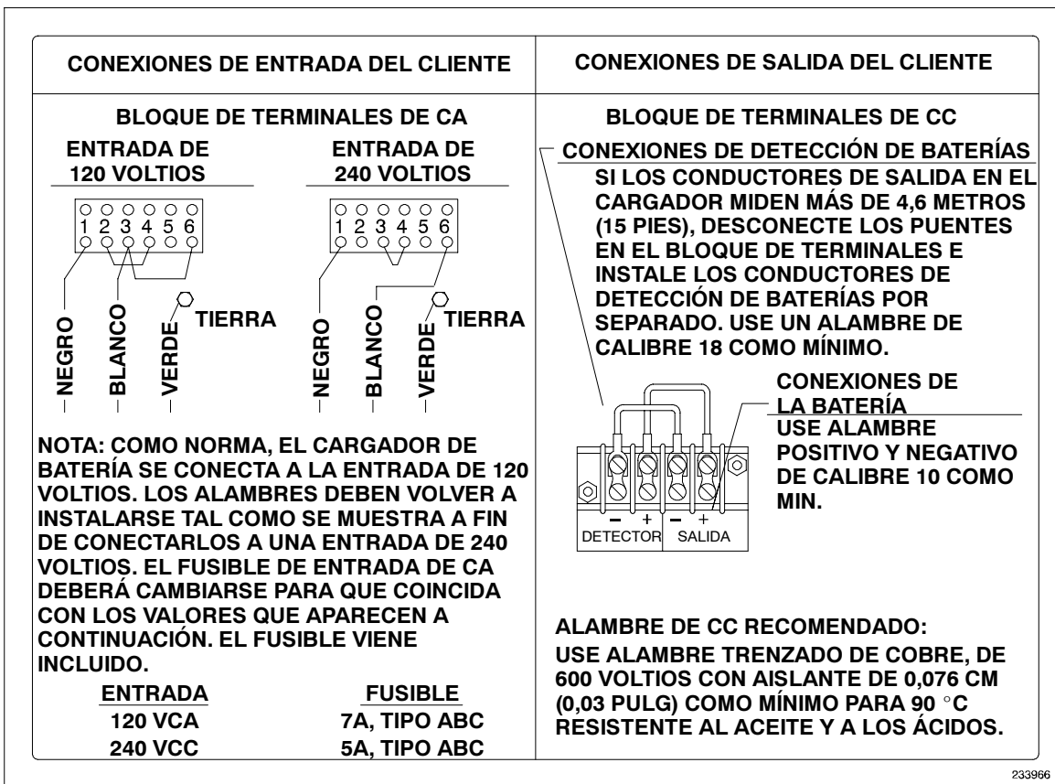
Figura 3. Conexiones de entrada de CA y de salida de CC del cliente
