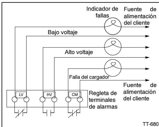
Figura 10. Conexiones del indicador de fallas del cliente
