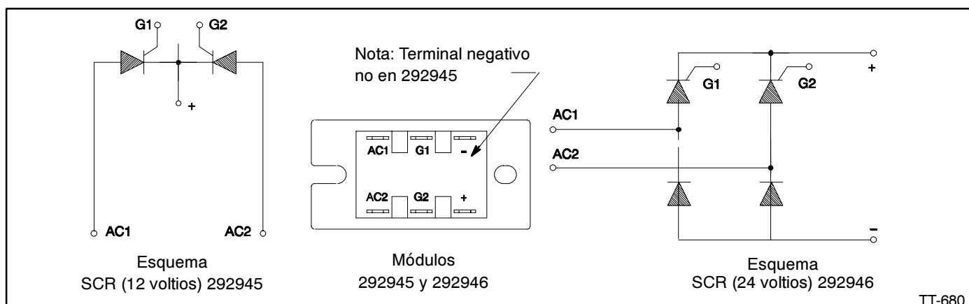
Figura 5. Módulos SCR
