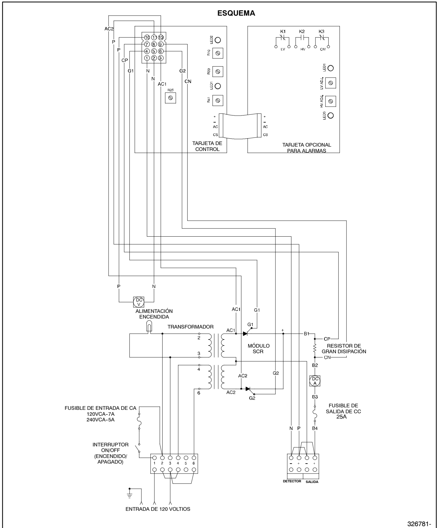
Diagrama de cableado, esquema, 326781A
