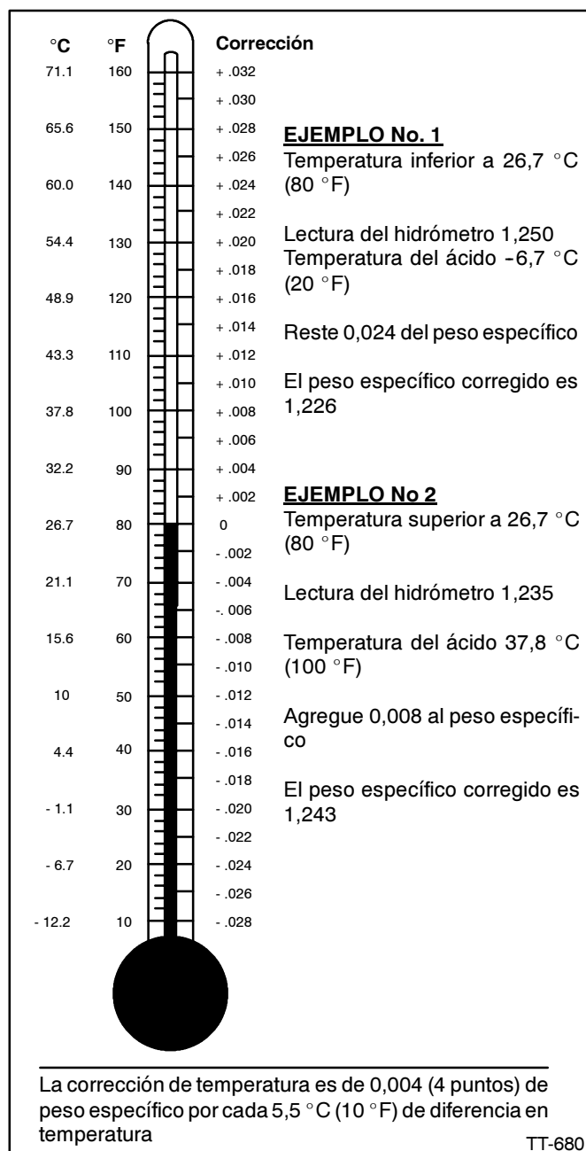
Figura 4. Corrección de la temperatura según el peso específico
