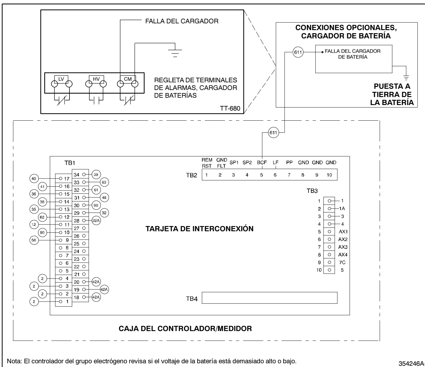
Figura 11. Conexiones del indicador de fallas A-352160 en la tarjeta de circuitos de control
