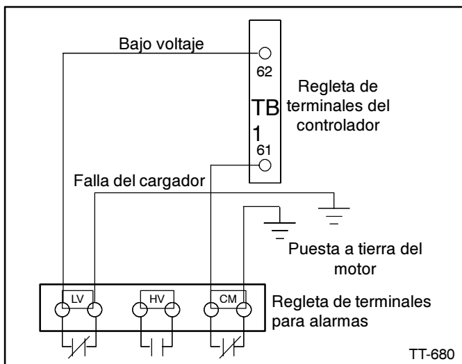
Figura 9. Conexiones del indicador de fallas en el controlador de microprocesador
